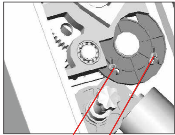
Vis de réglage horizontal de la lisse
